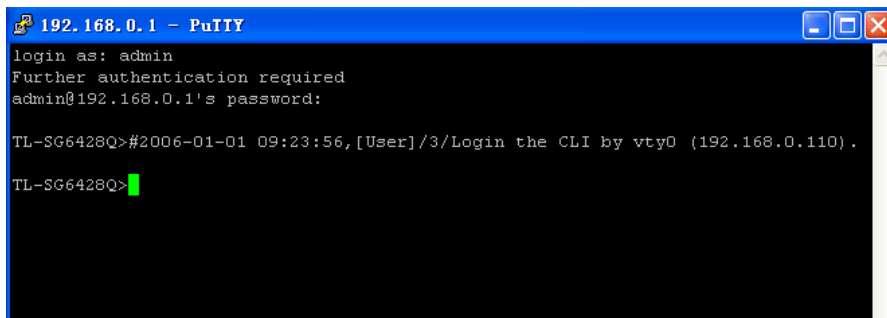
图 1-14 登录交换机
