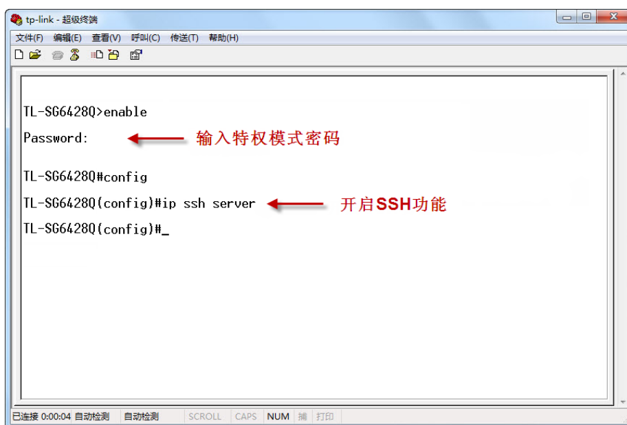
图 1-12 开启SSH功能
