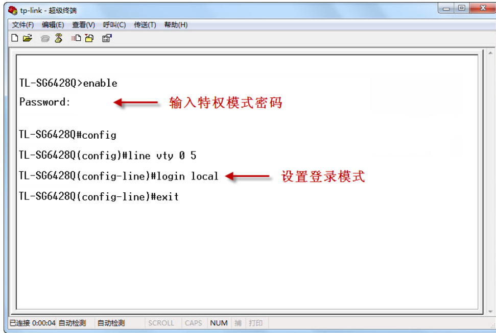
图 1-3 设置 login local 模式
